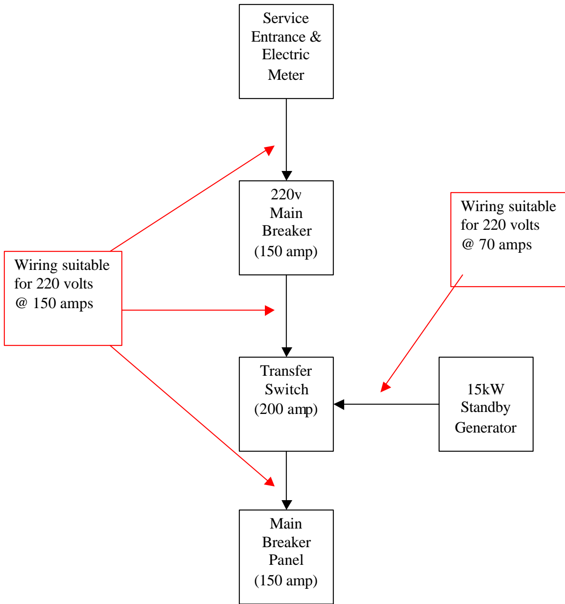
220v Wiring Schematic
